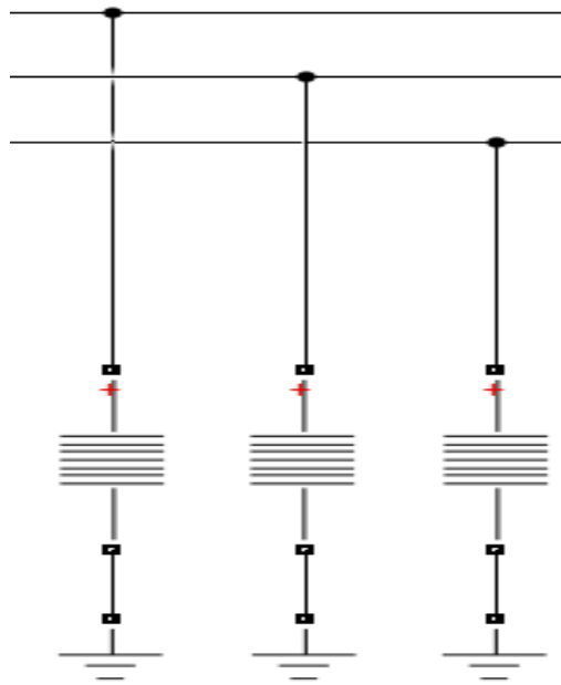
Fig. 8. SPD model
